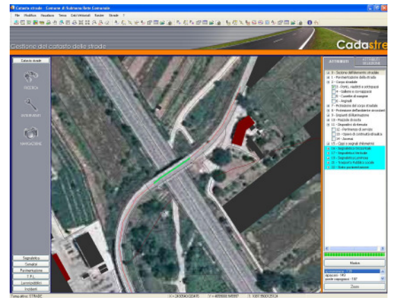
CADASTRE : gestione geo-database dei dati del catasto strade (DM 1/06/2001)
