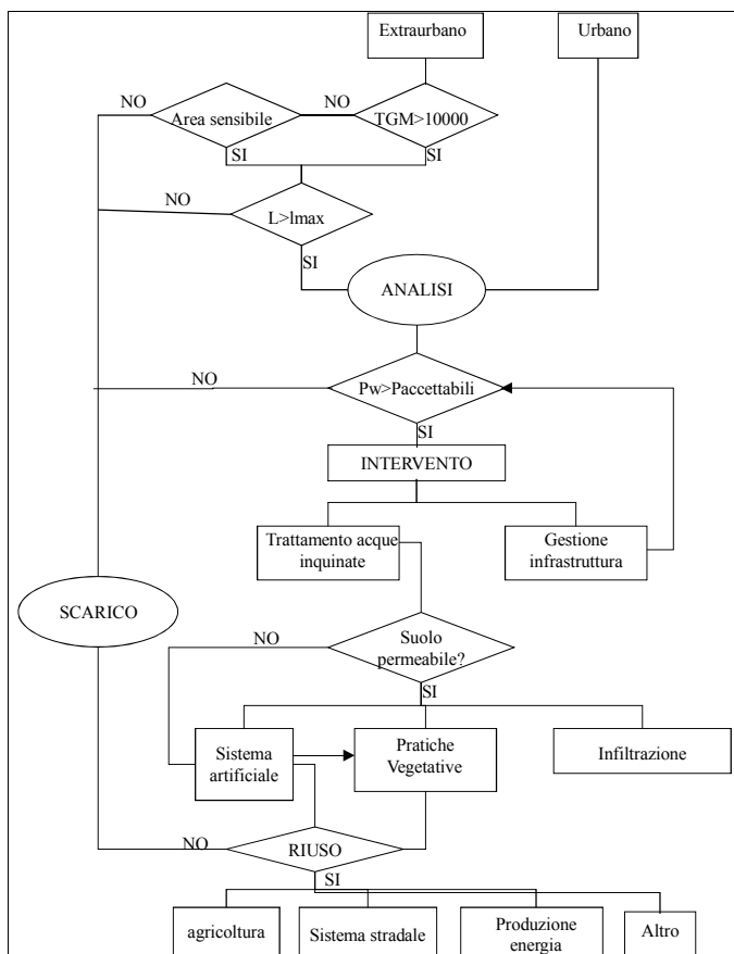
Flow-chart procedurale per la valutazione di impatto ambientale delle acque di ruscellamento stradale
